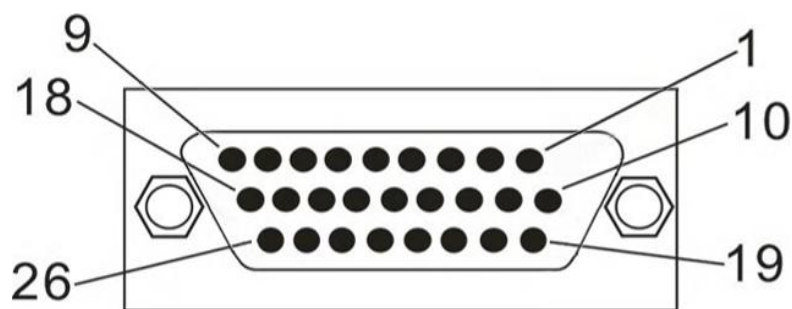
图 2.3 三排 DB26 母座
