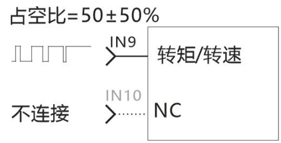
图 4.6.2 50% \pm 50\% 占空比控制
