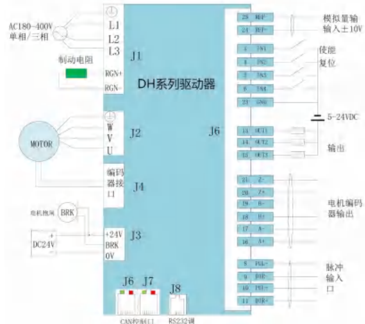
DH380V接线图
