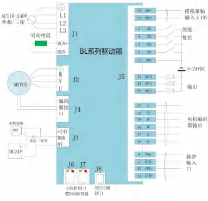
BL 220V接线图
