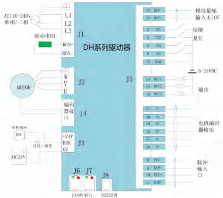
DH220V接线图
