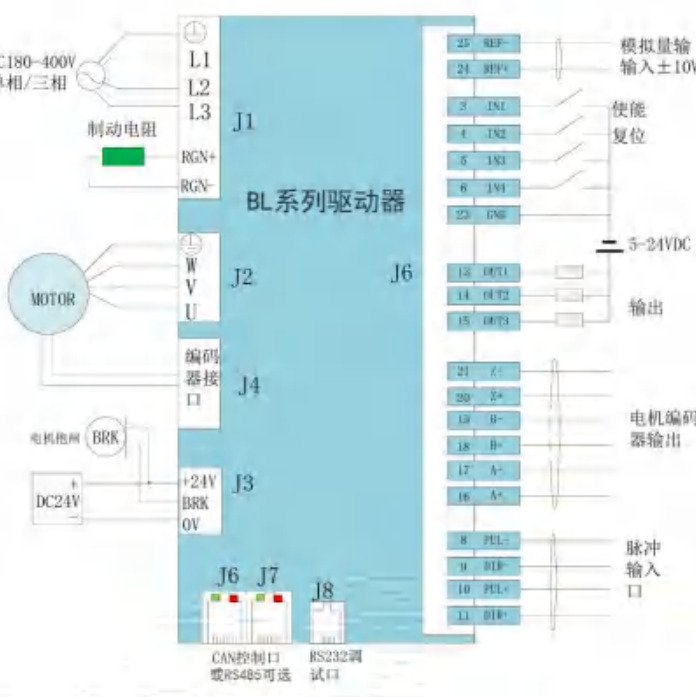
BL 380V接线图
