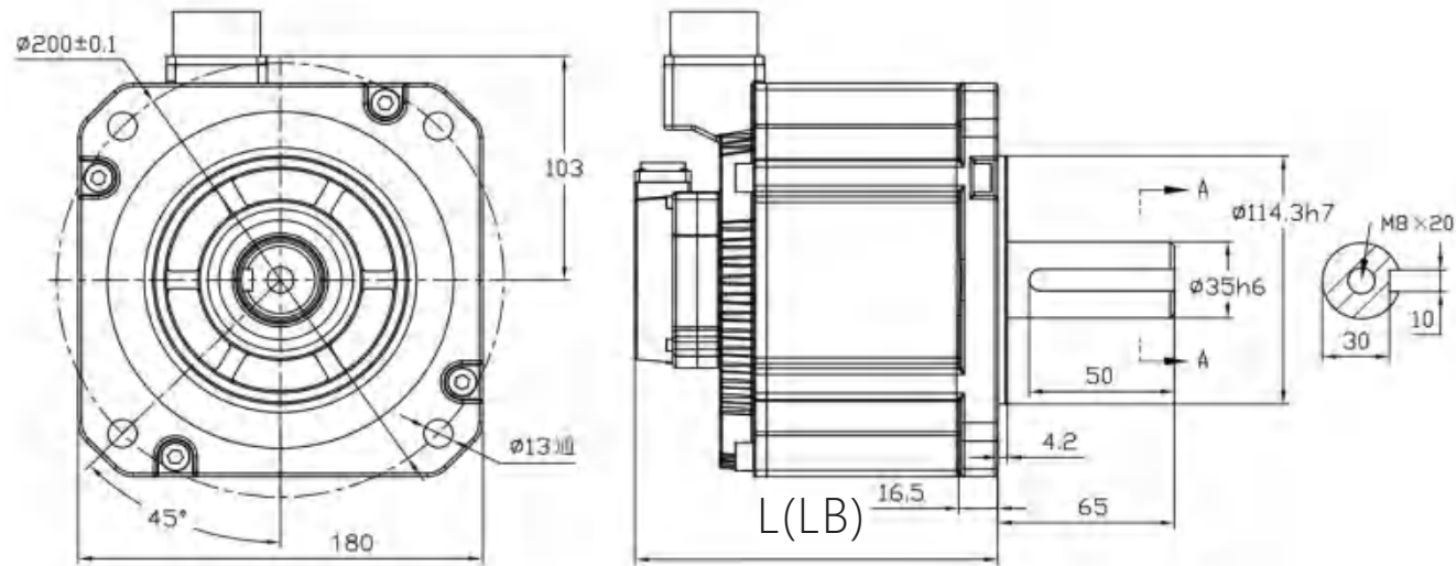
外形尺寸图
