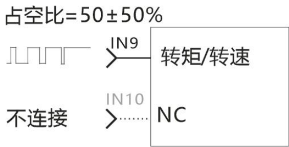
图 4.6.2 50%±50%占空比控制
