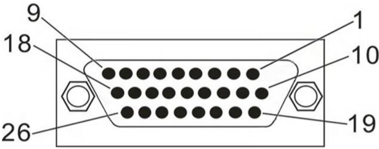
图 2.3 三排 DB26 母座
