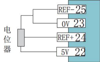
图3.3.3 内部电源模拟量输入接线
