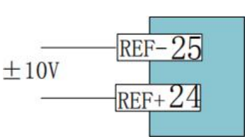
图3.3.2 外部电源模拟量输入接线
