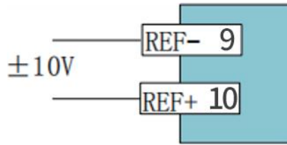
图 4.3.3 内部电源模拟量输入接线
