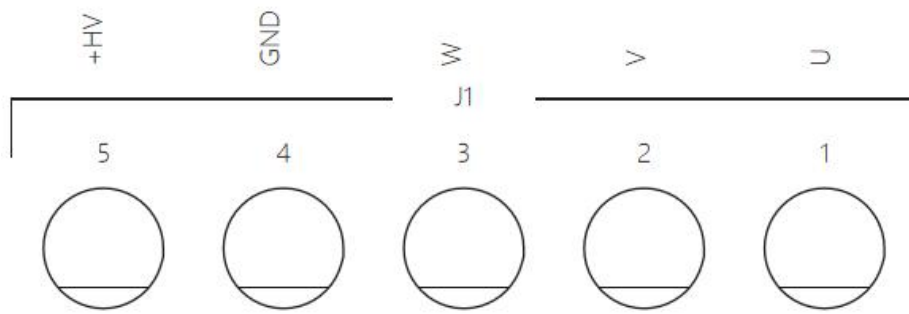
图 2.1 欧规端子
