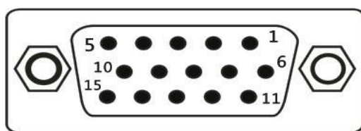
图 2.4.1 三排DB15母座
