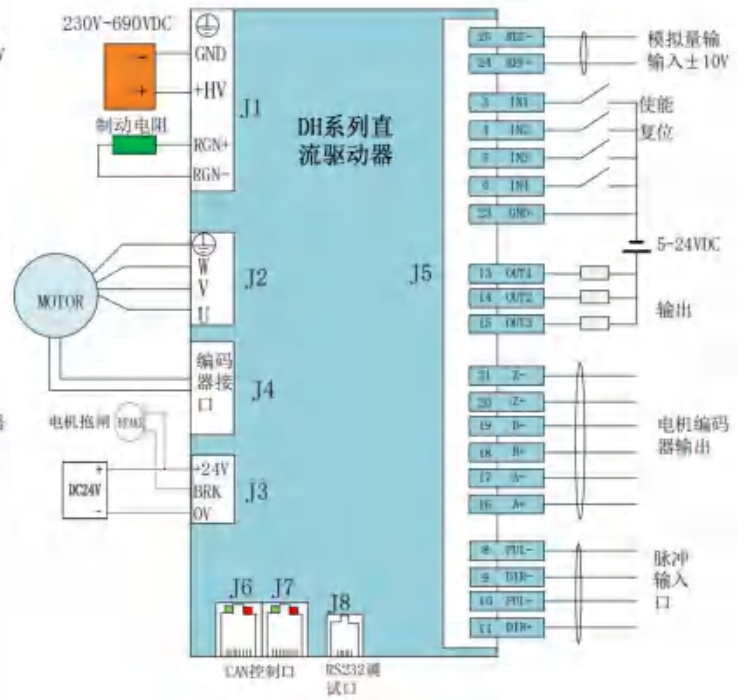
DH540V接线图
