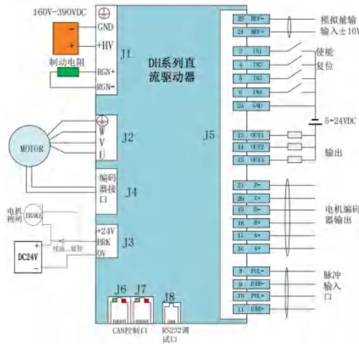
DH300V接线图
