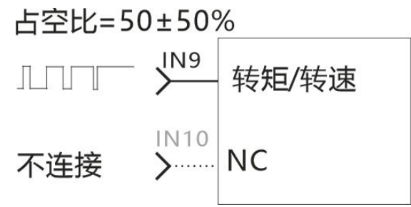
图 4.6.2 50%±50%占空比控制
