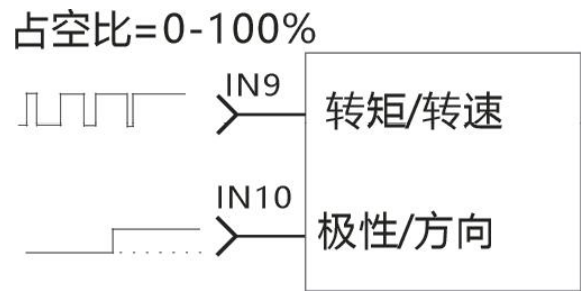
图 4.6.1 100%占空比+方向控制
