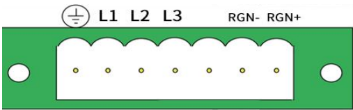
图2.1.2 欧规端子插座
