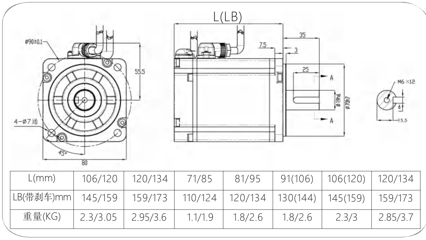
外形尺寸图
