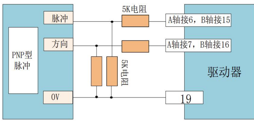
图 3.5.2 PNP脉冲输入图
