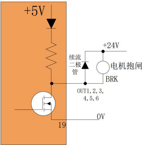
图 3.6.4 电机抱闸制动器外接电路
