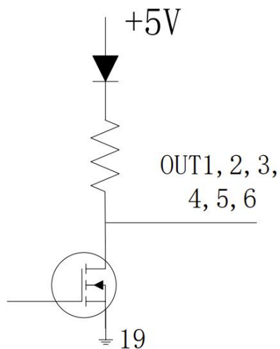
图 3.6.1 数字输出口硬件电路
