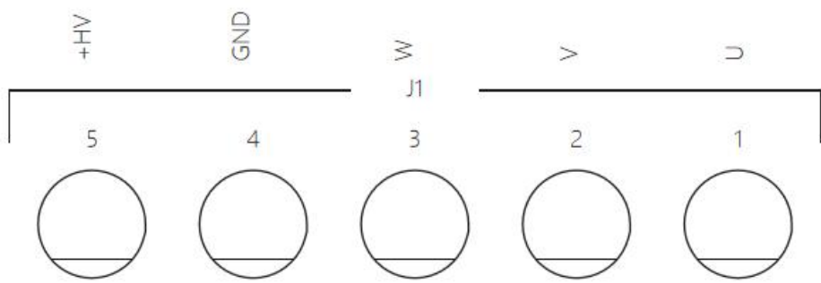
图 2.1 欧规端子
