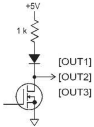
图 3.5 数字输出硬件电路
