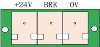
图2.3 欧规端子插座
