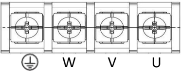
图2.2.2 栅栏端子插座
