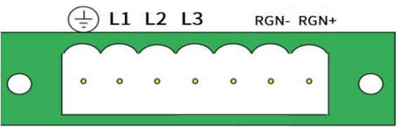
图2.1.2 欧规端子插座
