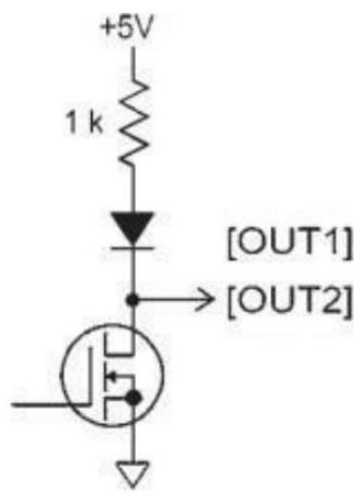
图 3.5 数字输出硬件电路
