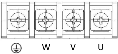
图2.2.2 栅栏端子插座
