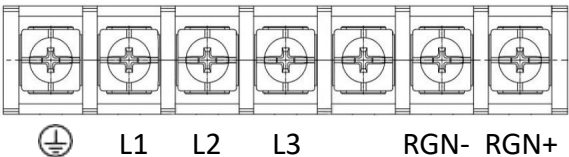
图2.1.2 栅栏端子插座
