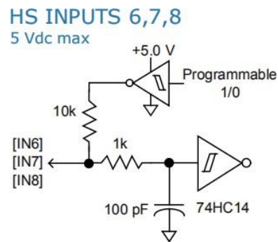
图 3.4.3 IN6,7,8内部硬件图图
