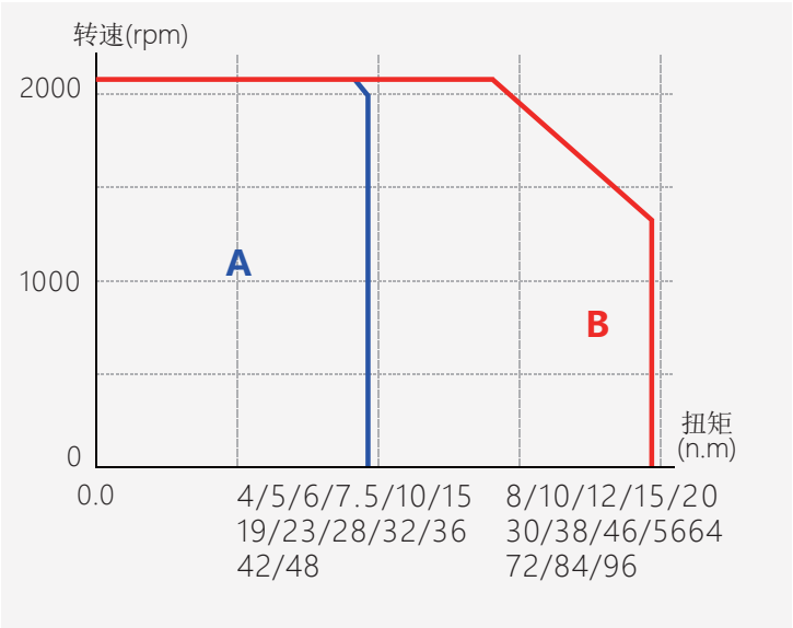
A:连续使用区域/Continuous Duty Zone B:瞬时使用区域/Intermittent Duty Zoue
