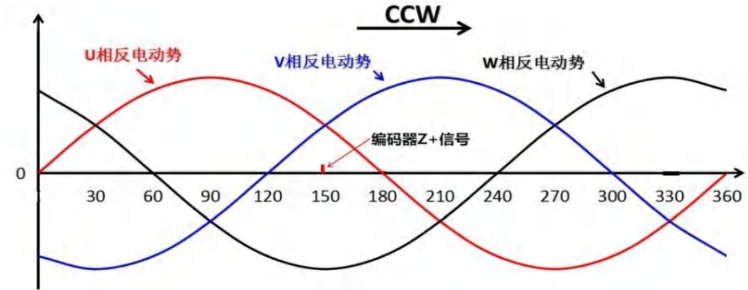
编码器零点与电机相位关系
