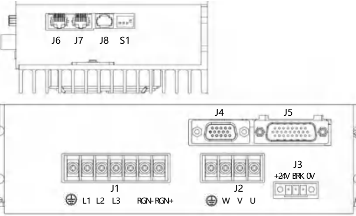
J3 内部24V输出端子(BL110/220V系列)
