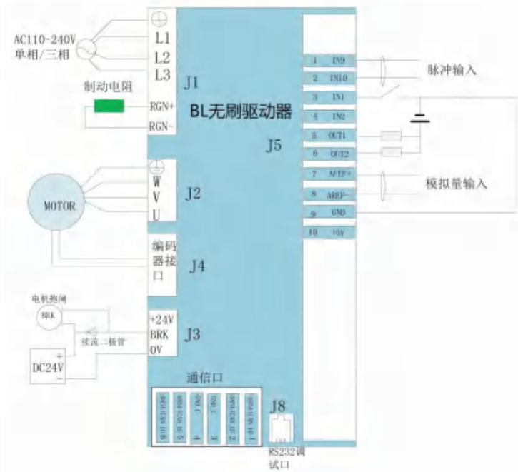
BL 110V/220V接线图
