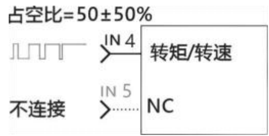
图4.5.2 50%±50%占空比控制
