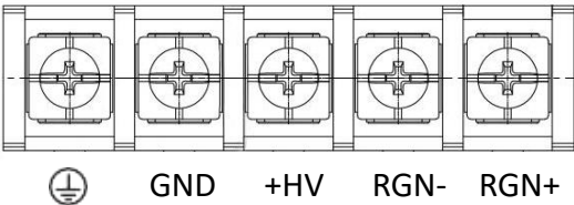
图2.1.2 栅栏端子插座
