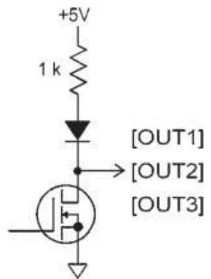
图 3.5 数字输出硬件电路
